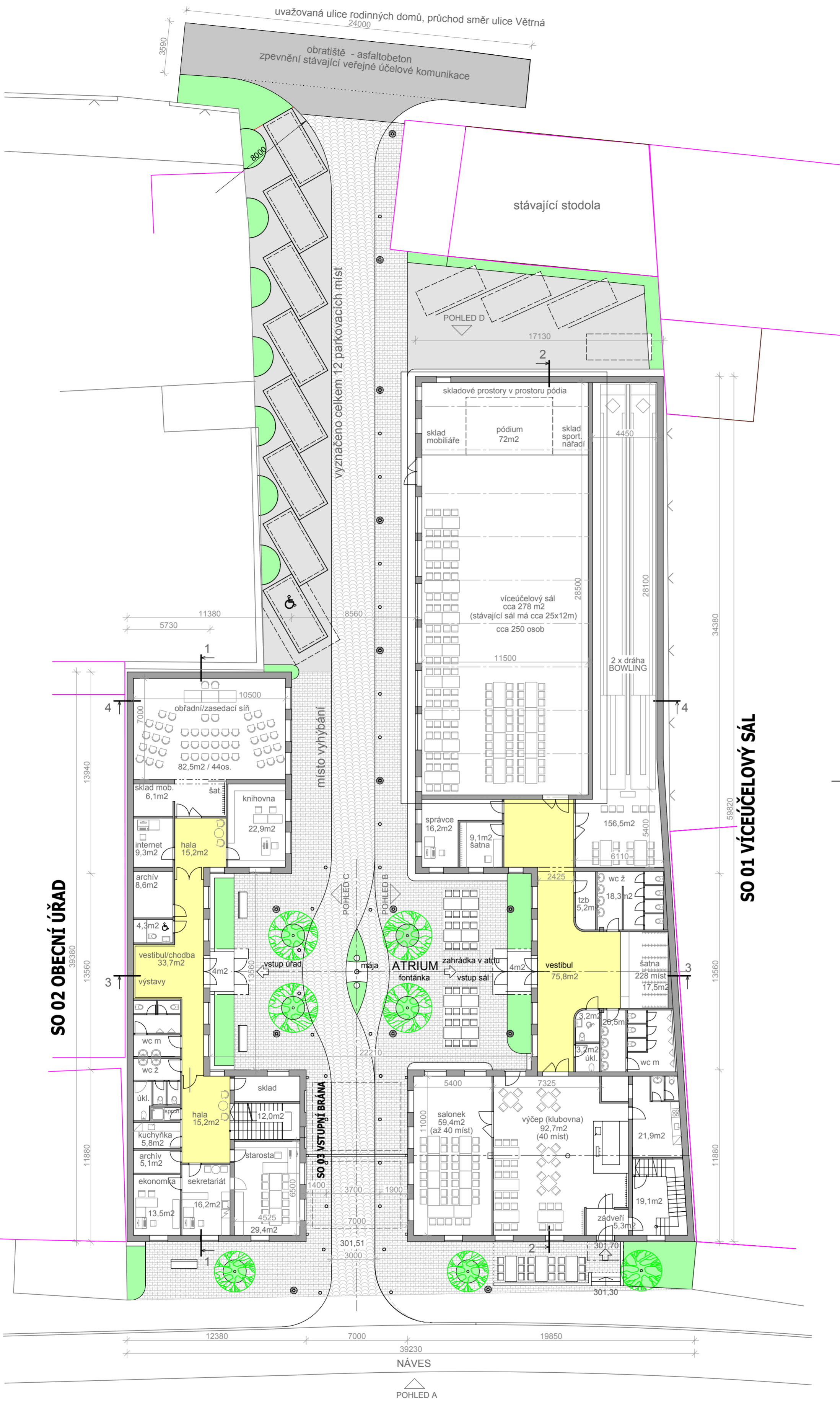
PŮDORYS 1.NP
